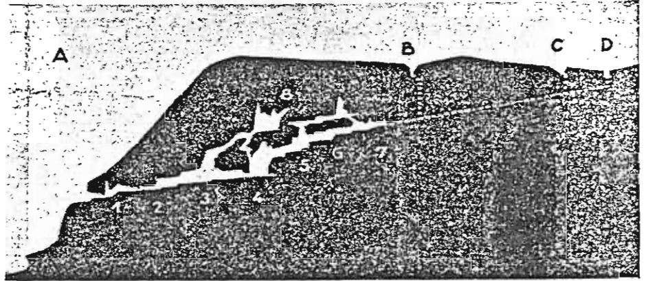
Vaux, établi par M. NUFFER, le chef de l'expédition, un profil schématisé du plateau dans lequel se trouve la rivière souterraine du Cul-de-Vaux. Il a le mérite d'éclaircir le processus de transformation de cette rivière en grand égout collecteur.
